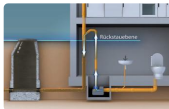
Bild 1: Rückstauabsperrung
